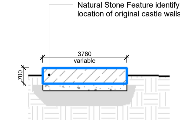
4 STONE PAVER DETAIL SCALE: 1 : 100
